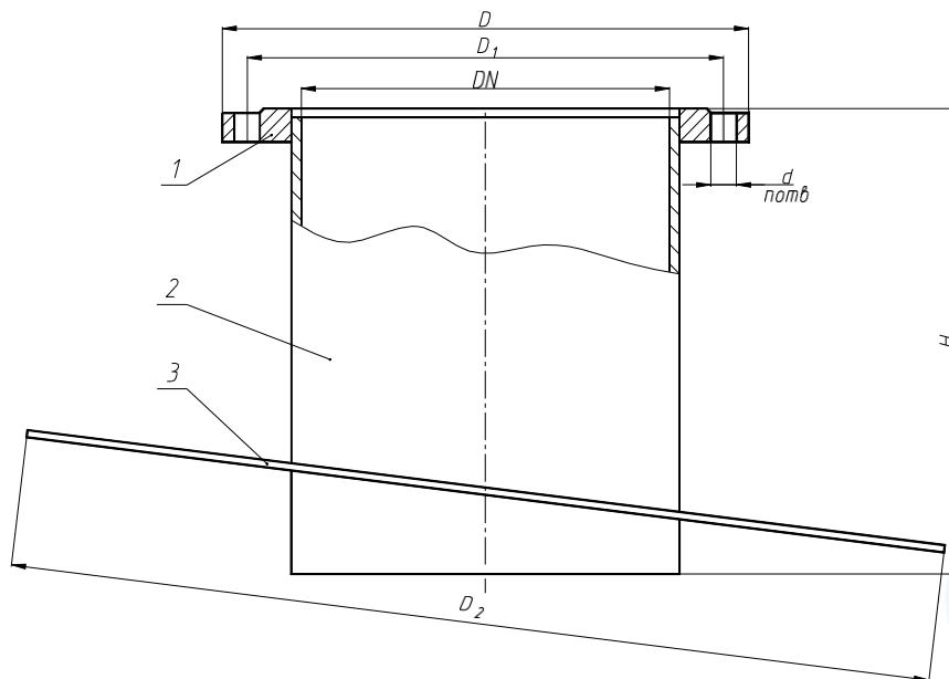
1 – фланец, 2 – труба, 3 – усиливающая накладка.
