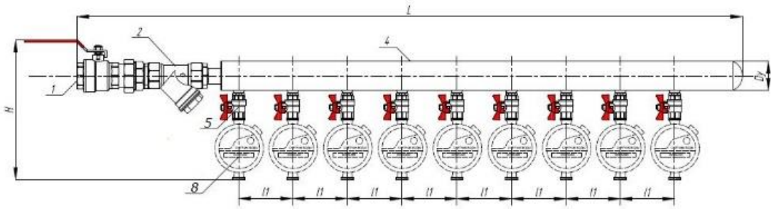
Коллекторный узел ХВС и ГВС без регулятора (Вариант 5)
