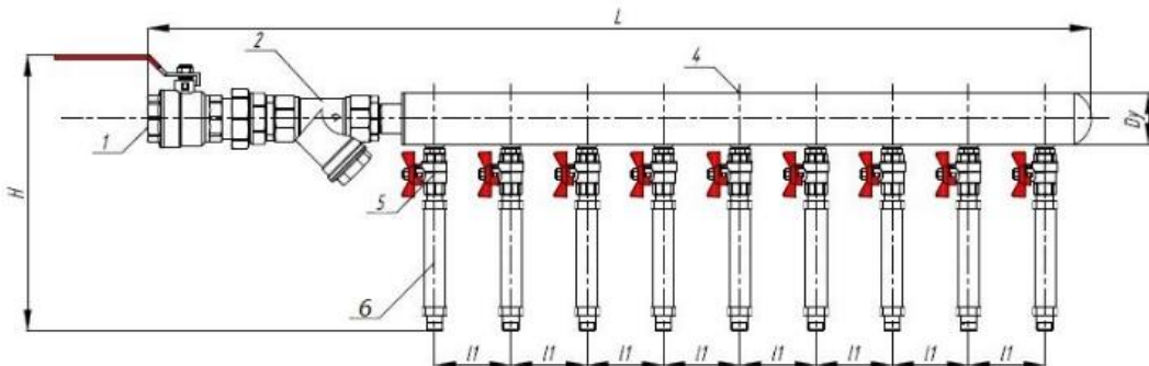
Коллекторный узел ХВС и ГВС с индивидуальным регулятором (Вариант 3)
