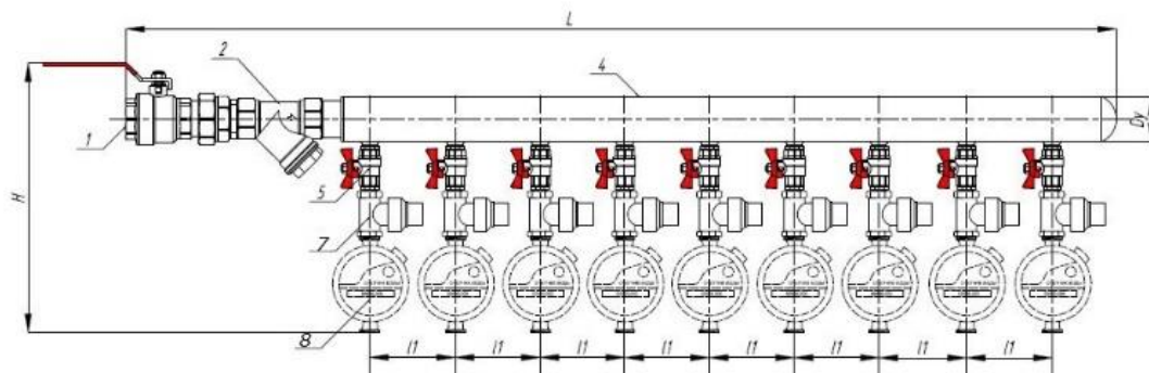
Коллекторный узел ХВС и ГВС с индивидуальным регулятором и счетчиками (Вариант 4)
