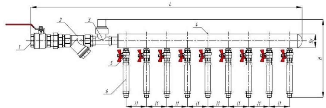
Коллекторный узел ХВС и ГВС с общим регулятором и счетчиками (Вариант 2)
