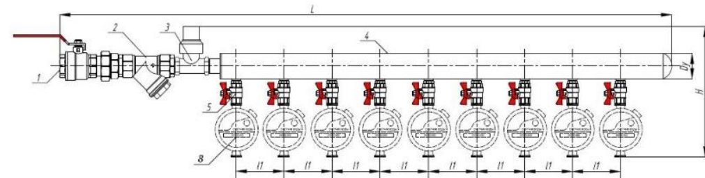
Коллекторный узел ХВС и ГВС без регулятора, со счетчиками (Вариант 6)
